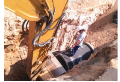
Orhanlı Mahallesi Sabancı Caddesi Ø1000 mm Yağmursuyu Hattı Çalışması
